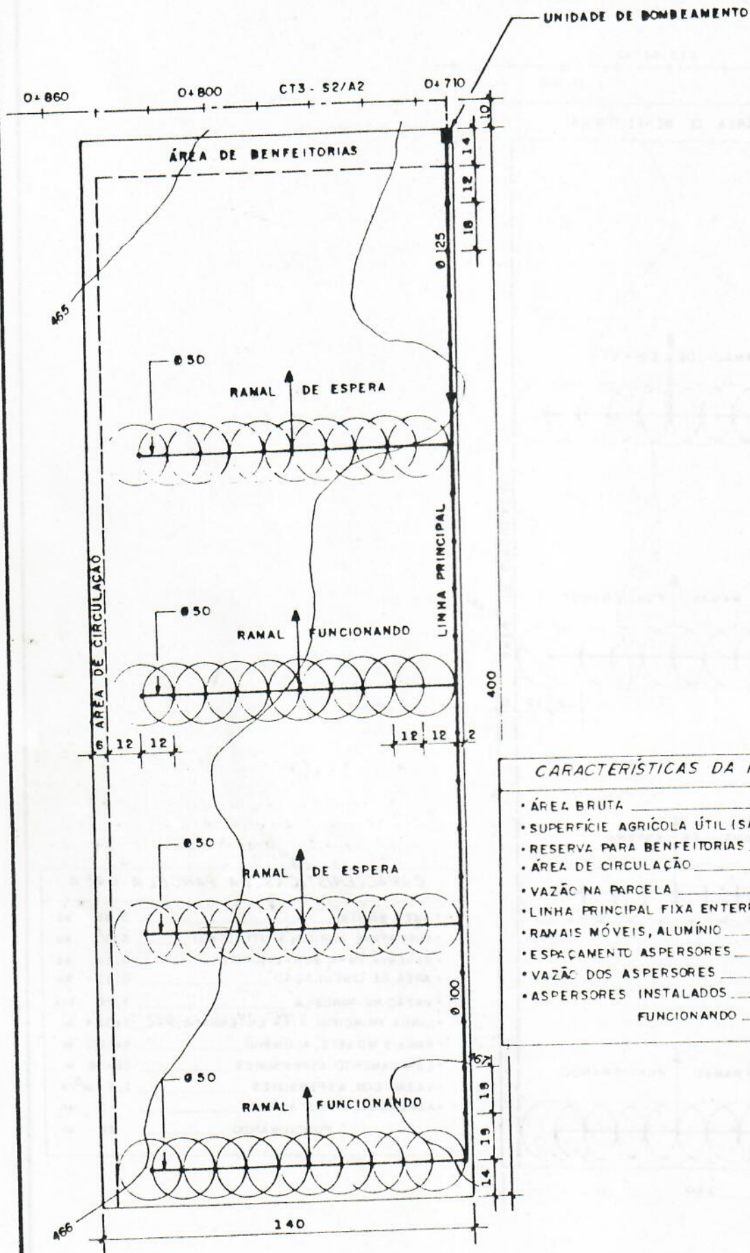
Fig. 26 REDE PARCELAR
