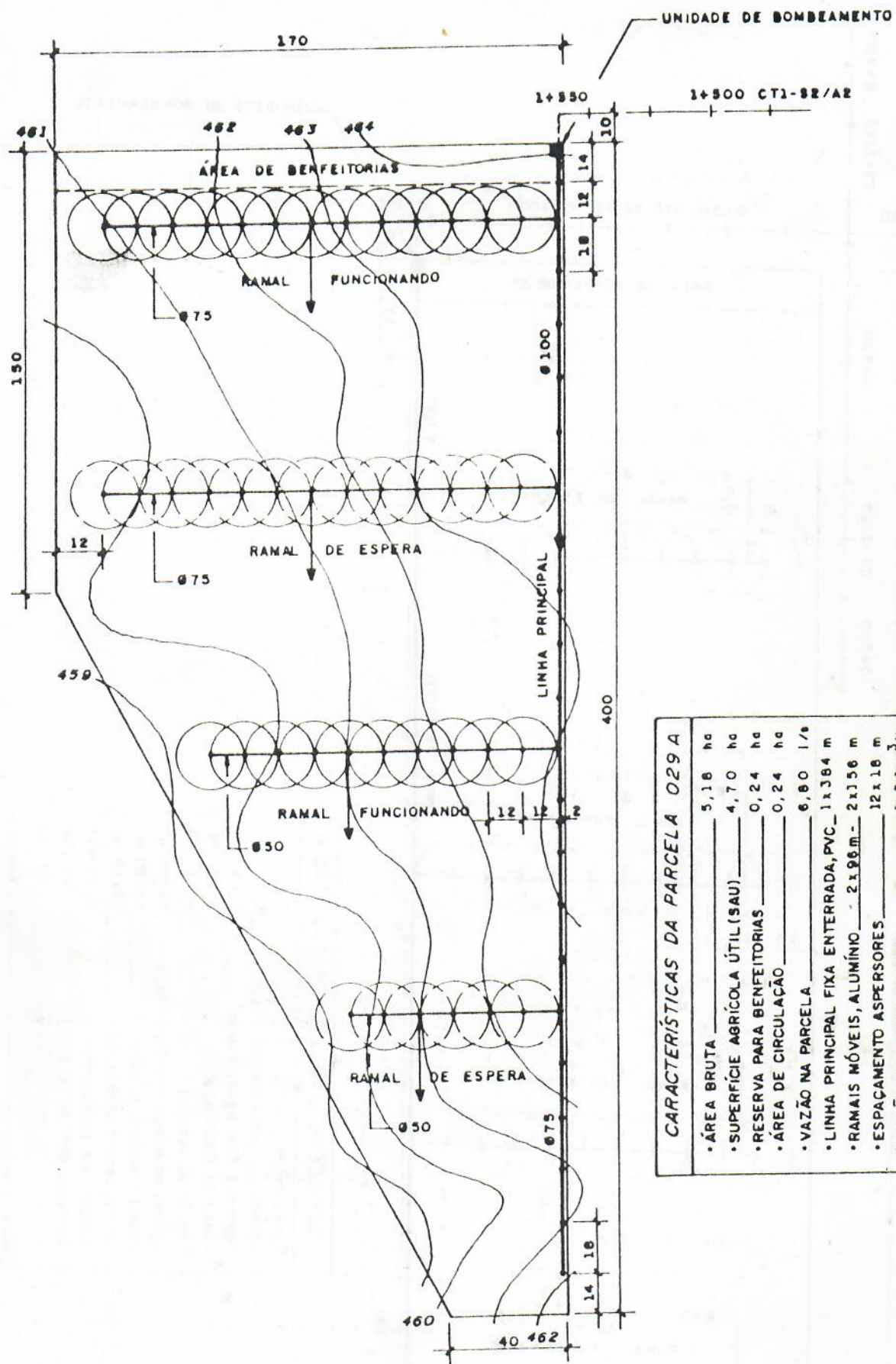
Fig. 29 REDE PARCELAR
