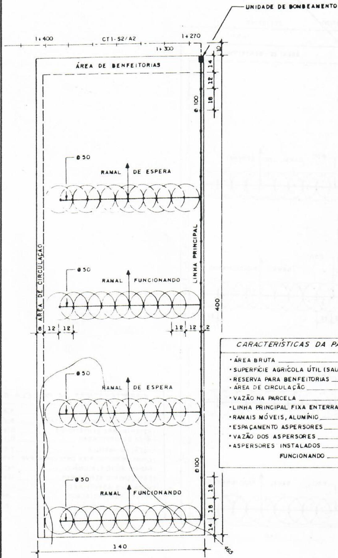
Fig. 25 REDE PARCELAR
