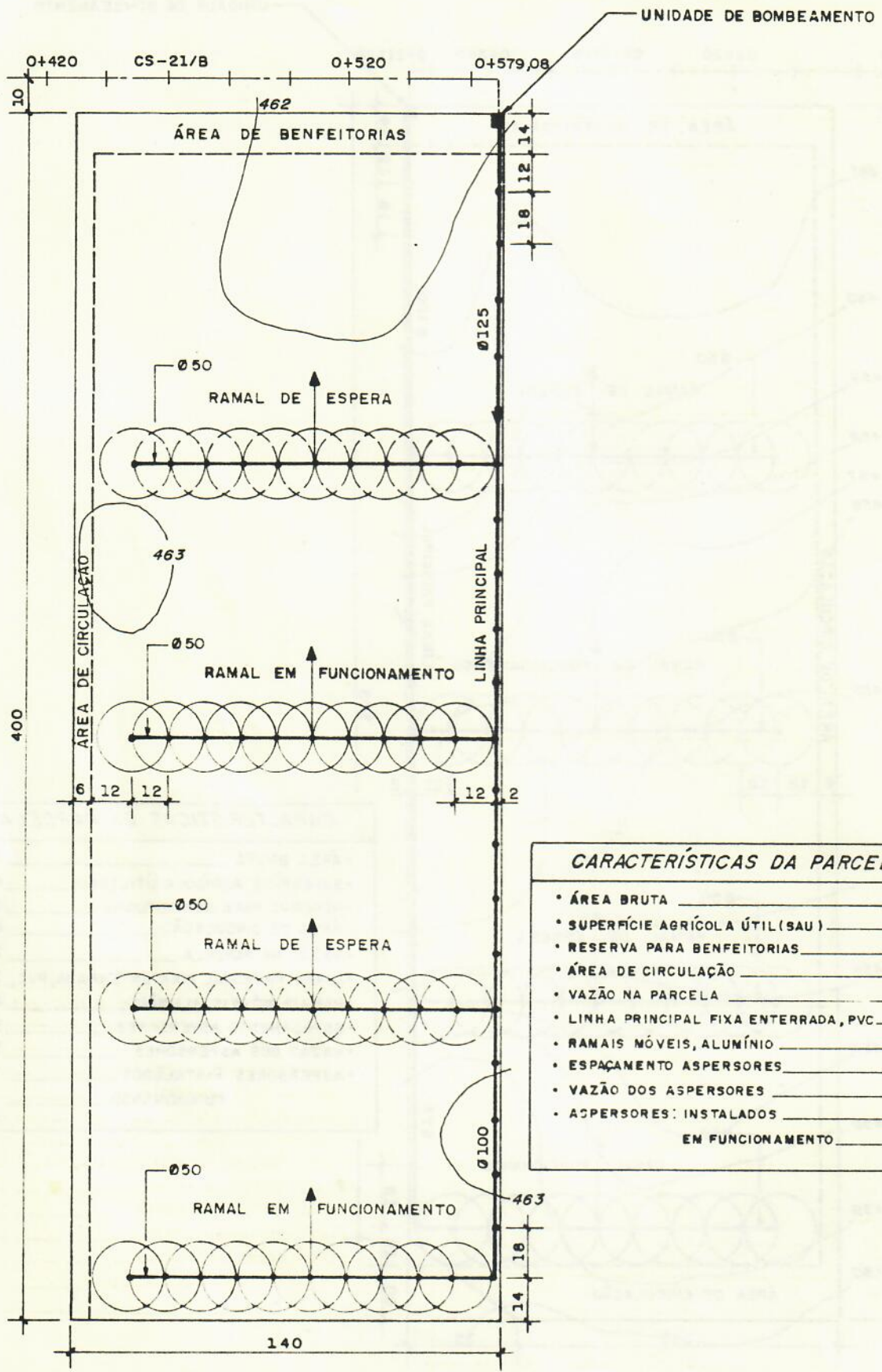
REDE PARCELAR
