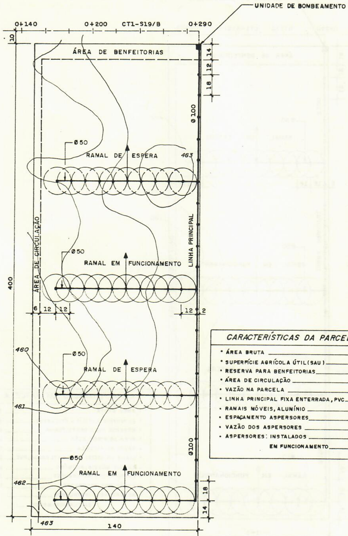
REDE PARCELAR
