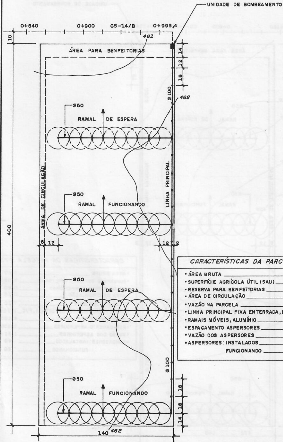
REDE PARCELAR
