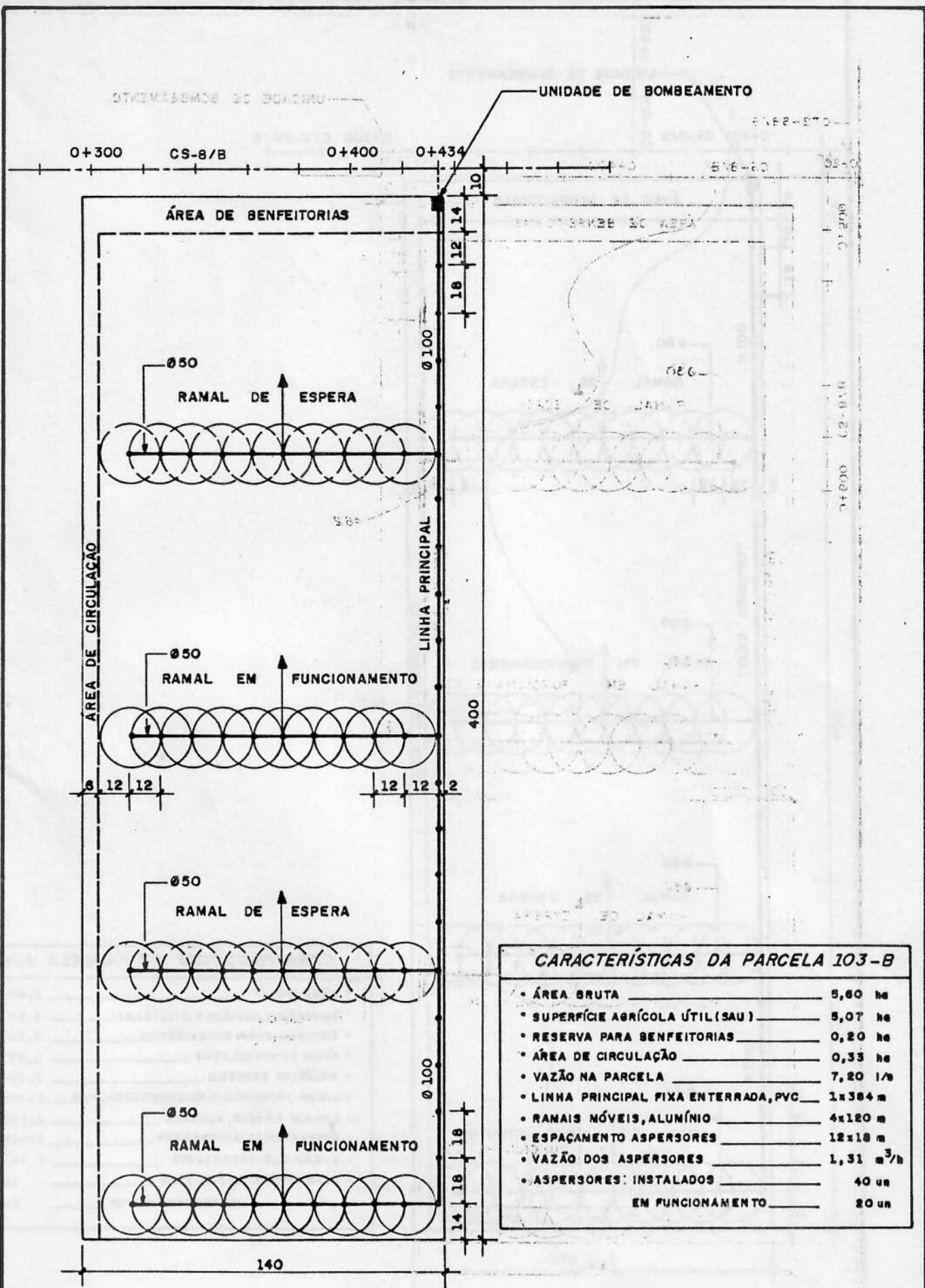
REDE PARCELAR
