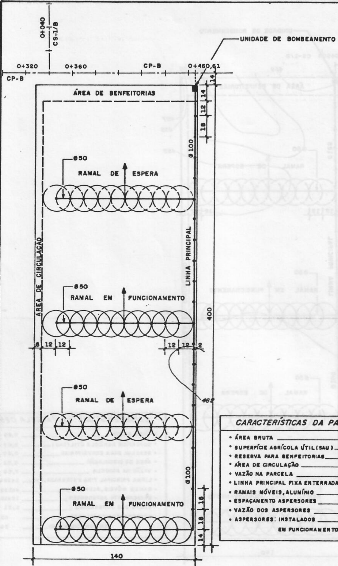
REDE PARCELAR
